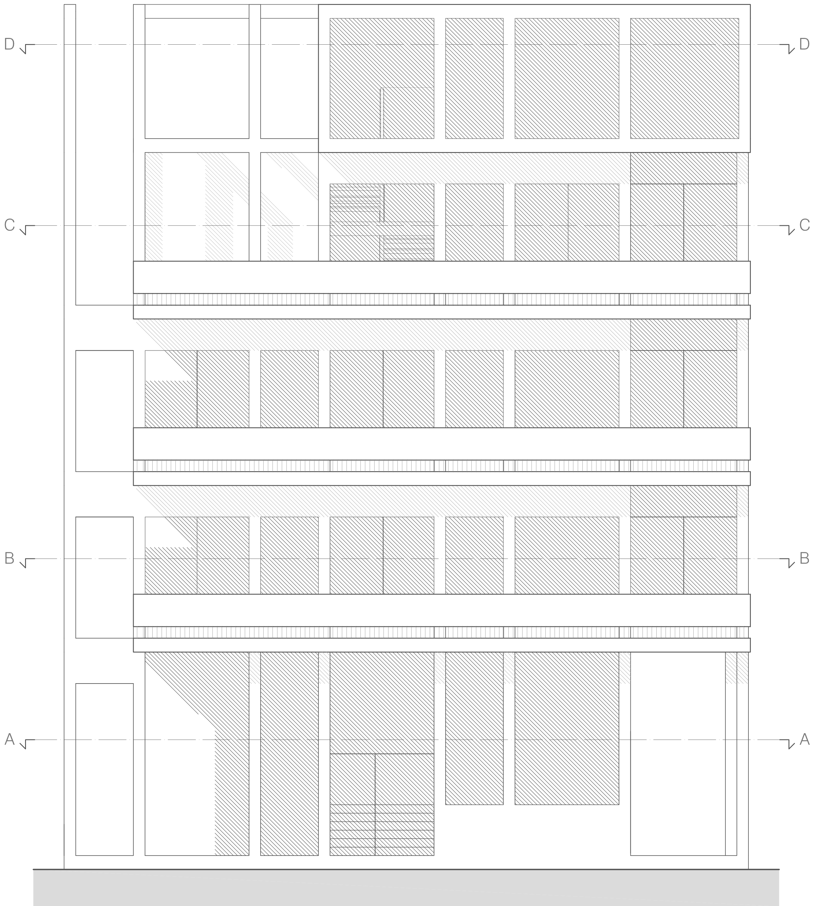
Prospetto Sud
