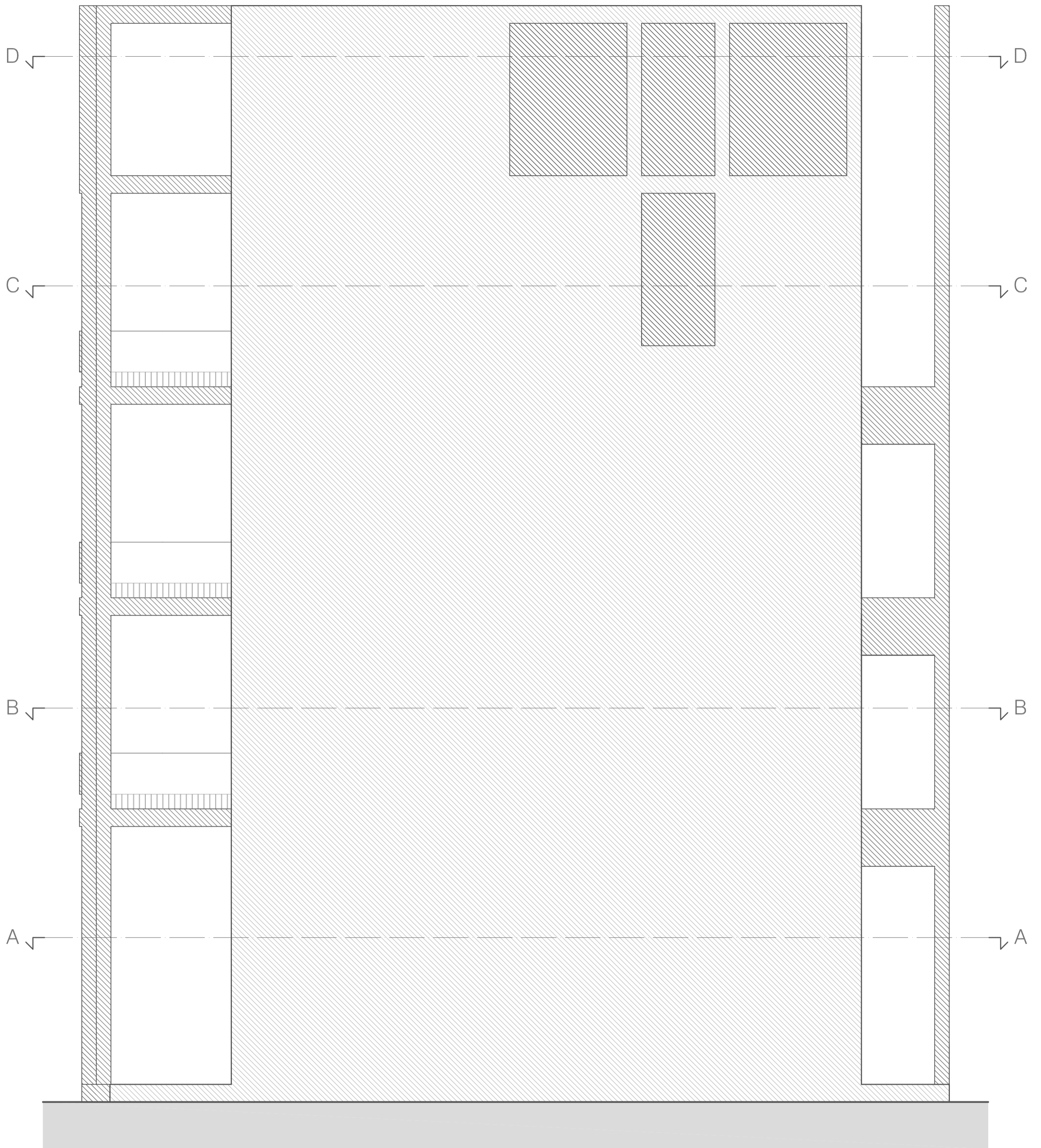
Prospetto Nord
